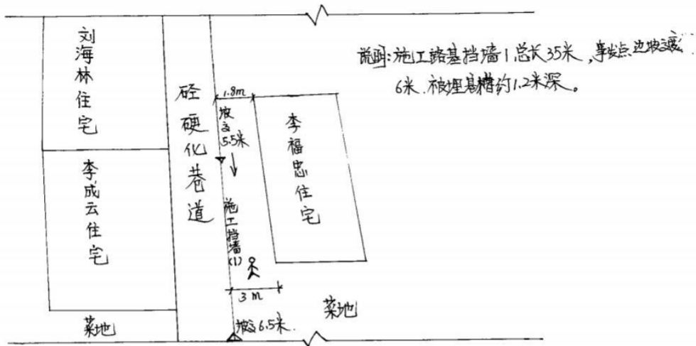
羊沙镇大草滩村路基防护工程“7.06”事故点平面示意图
